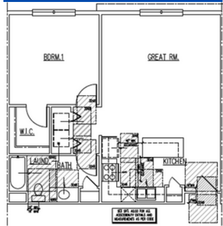
UNIT PLAN 1BR-A
